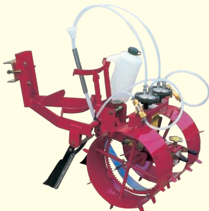
MI-408 (ティラー用) 2条ちどり(間欠)注入式
