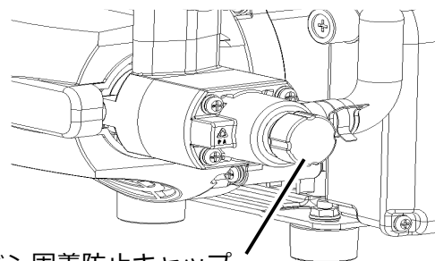
ベン固着防止キャップ
