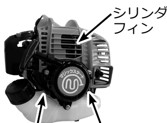
冷却風取出口 (格子部)
