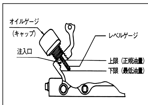
オイル点検
