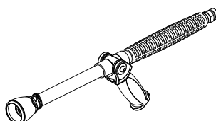
タービンランス組立 /1 個 MKW0730EFS (665578) MKW0536EFS (666008) MKW0730EFS (666323)
