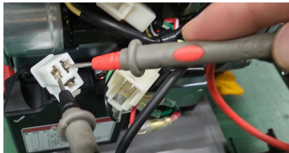
サーモスタット端子
