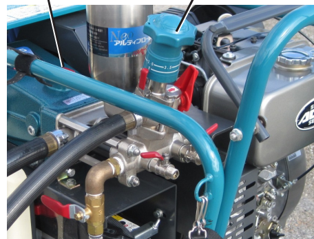
噴霧用ポンプ 調圧ダイヤル
