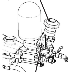
調圧弁ハンドル 始動位置
