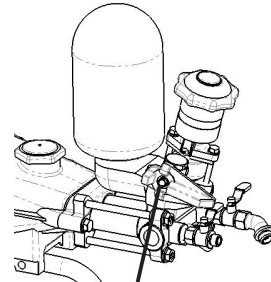
調圧弁ハンドル 加圧位置
