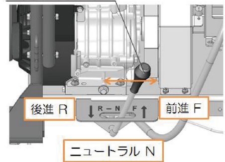
前後進シフトレバー
