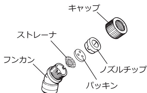
【ワイドノズル1頭口】
