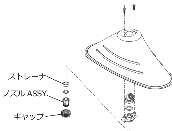
【カバー付き除草ノズル】
