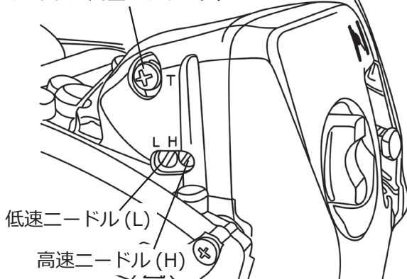
アイドル調整スクリュー(T)
