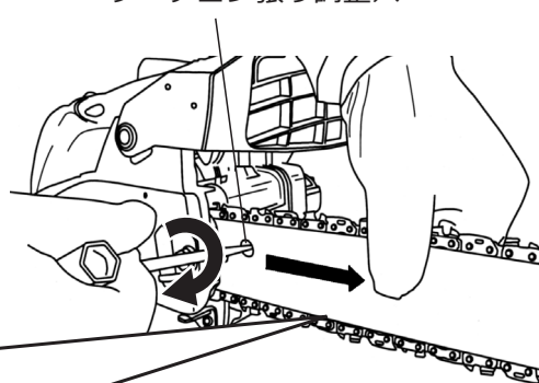
ソーチェーン張り調整穴
