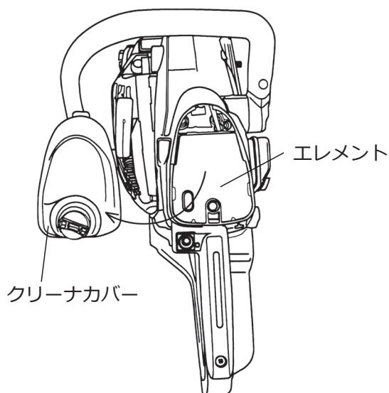
ノブを左に回しクリーナカバーを取り外します
