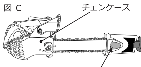
フックがチェーンケース側に向くように取付ける
