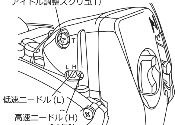
アイドル調整スクリュー(T)
