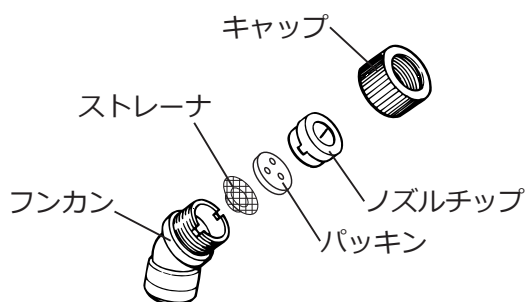
【ワイドノズル1頭口】
