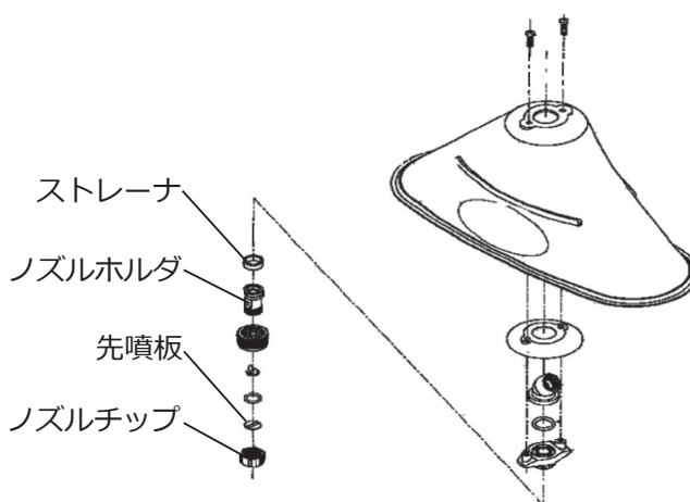
【カバー付き除草ノズル】
