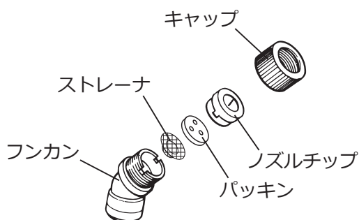
【ワイドノズル1頭口】
