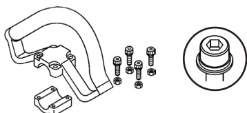
ループハンドル /1個 (227816)
