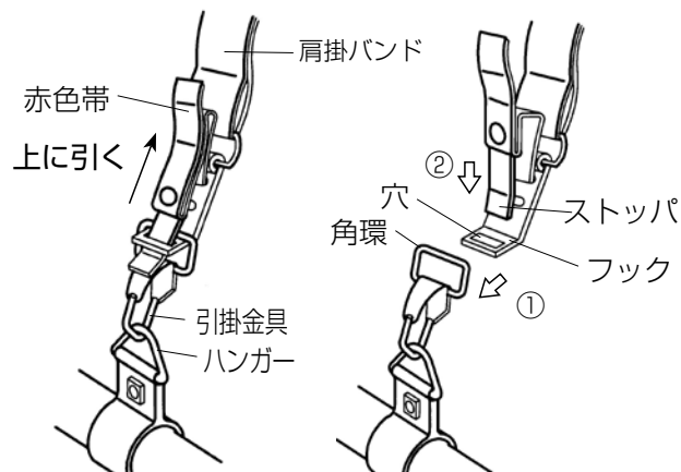
緊急離脱装置
