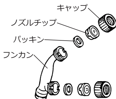
【2 頭口ノズル】
