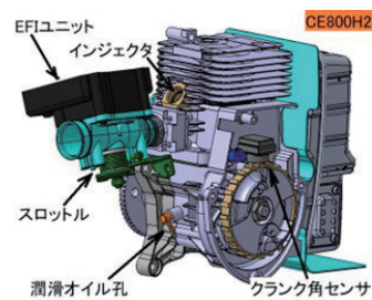
エンジン構造図
