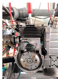
2ストローク水素エンジン
