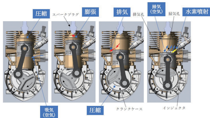
2ストローク水素エンジン燃焼のしくみ
