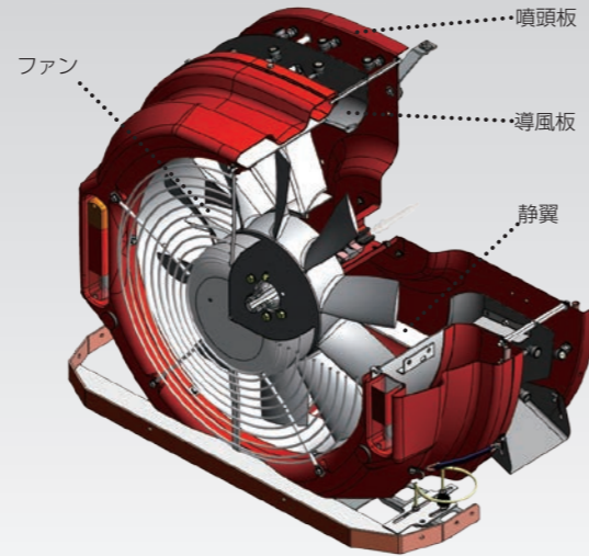
■ファン部イメージ図
