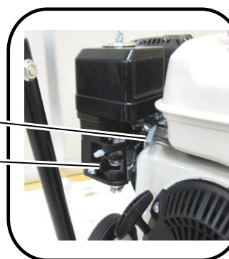
燃料コック
