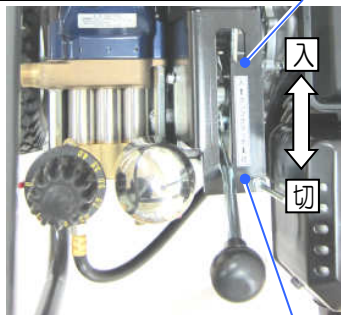
ポンプクラッチレバー「切」
