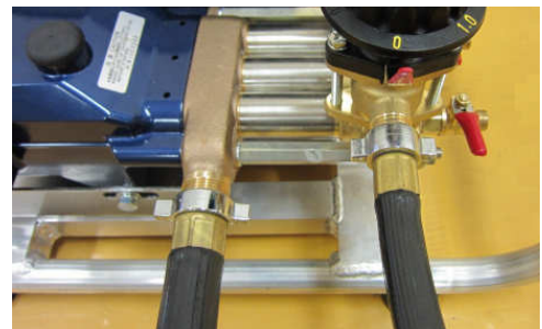
吸水ホース
