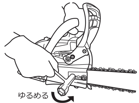
ソーチェン張り調整穴
