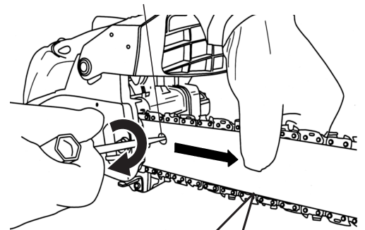
ソーチェン張り調整穴
