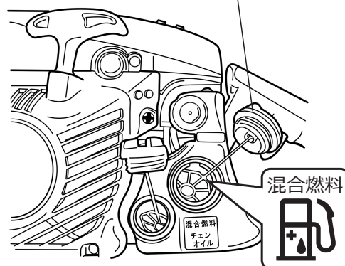
燃料キャップ(オレンジ)
