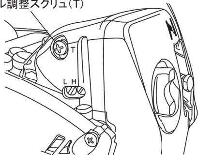
アイドル調整スクリュ(T)
