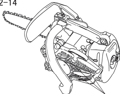
冷却空気取入口
