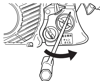
燃料キャップ (オレンジ)
