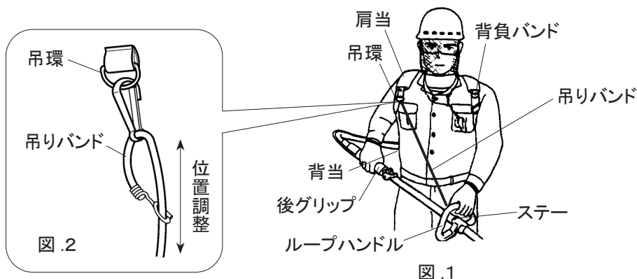
【装着図】
