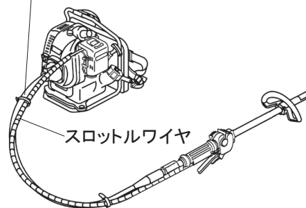
フレキシブルシャフト
