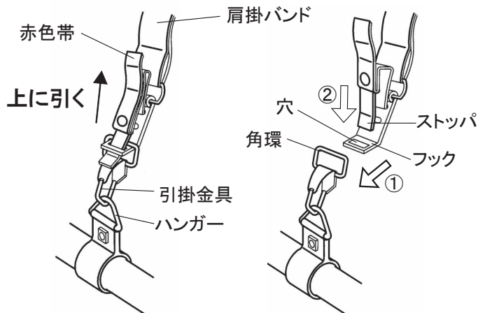
緊急離脱装置 図.3
