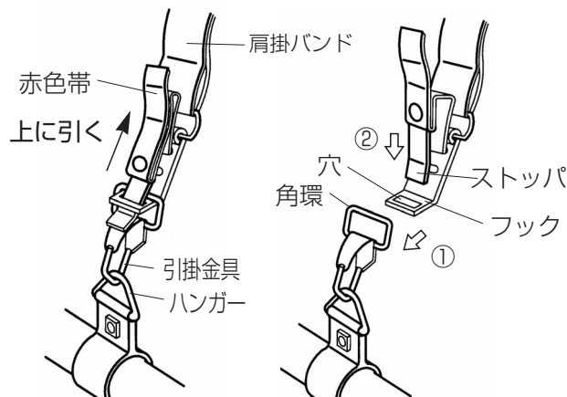
緊急離脱装置 図3
