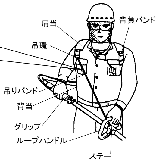
【装着図】
