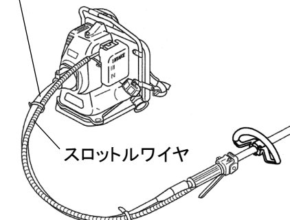
フレキシブルシャフト
